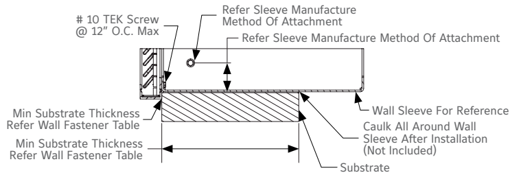
DETAIL CY N.T.S.
