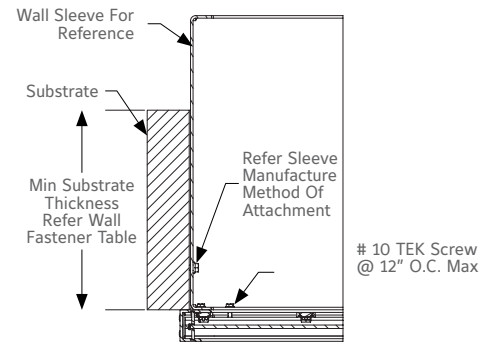
DETAIL CV N.T.S.
