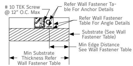
DETAIL BN N.T.S.
