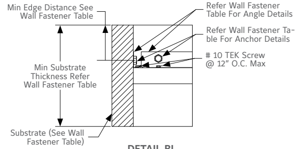
DETAIL BL N.T.S.
