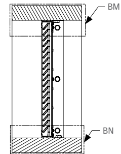
SECTION BJ-BJ N.T.S.
