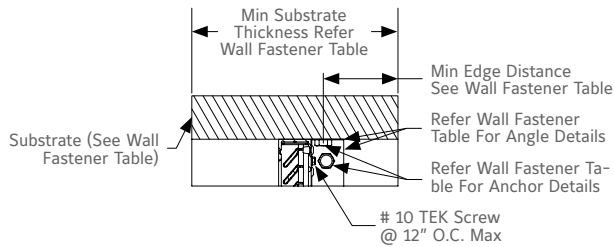
DETAIL BM N.T.S.
