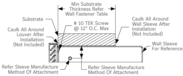
DETAIL CW N.T.S.
