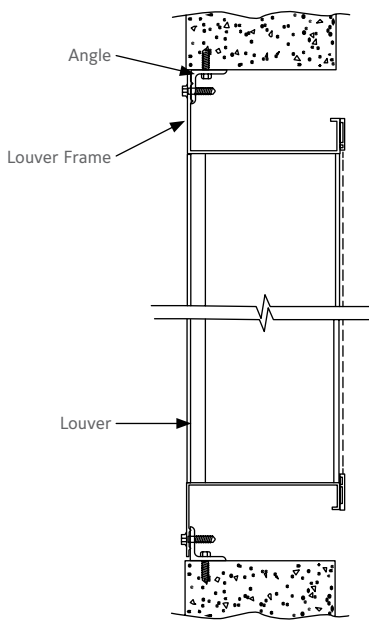
ANGLE SUBFRAME (OPTIONAL)
